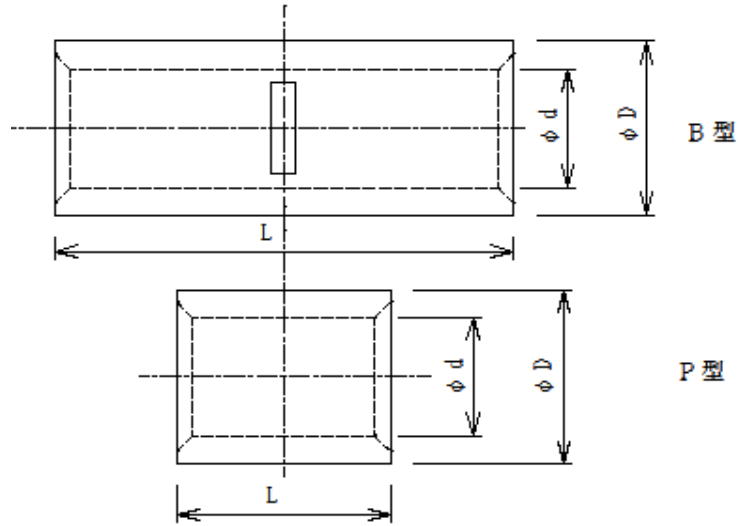
裸圧着スリーブ(B型/P型)
